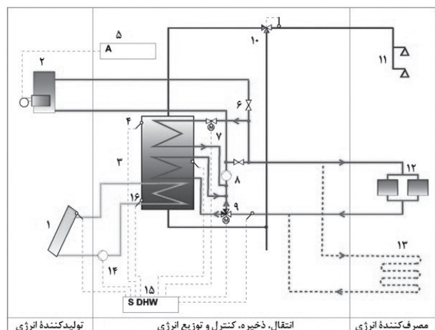
تصویر ۱- مدار شماتیک یک سامانه ترکیبی خورشیدی برای تأمین آب‌گرم و گرمایش محیط.
