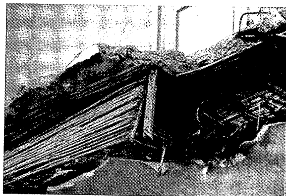
تصویر ۷- قالب بتن با نی در پردیس مرکزی دانشگاه تهران
