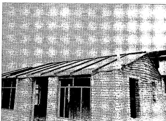
تصویر ۵- صفحات بافته شده از نی به عنوان جزئی از سقف، قالب بتن و عایق حرارتی
